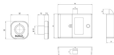
Padrão de Instalação em Portas
