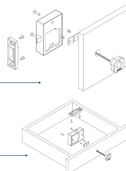
Padrão de Instalação em Portas
