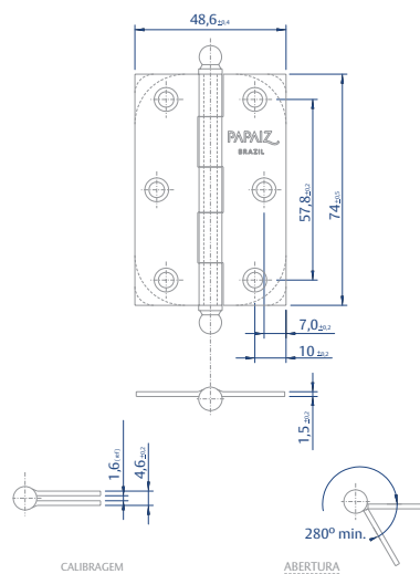
Desenho Dobradiças 1300 Aço 3"
