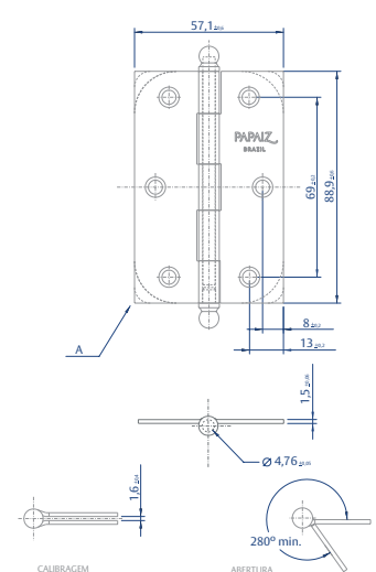
Desenho Dobradiças 1300 Aço 3 1/2"
