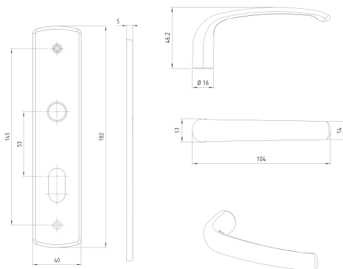
ESPELHO E230, E234 e E235
